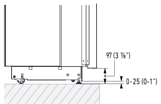
PLINTH SIZE
