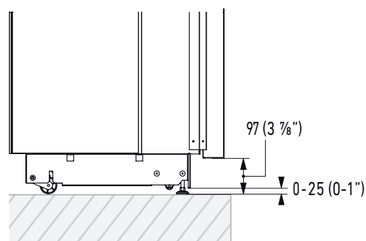
PLINTH SIZE
