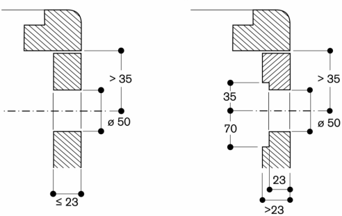
Montage bedieningsknop, vlak geïntegreerde inbouw
