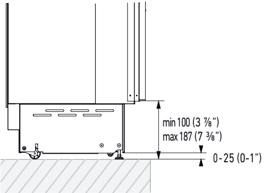
PLINTH SIZE
