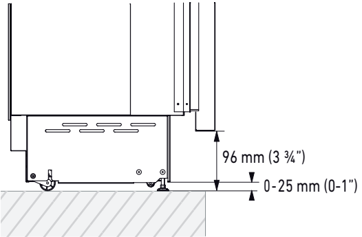
PLINTH SIZE
