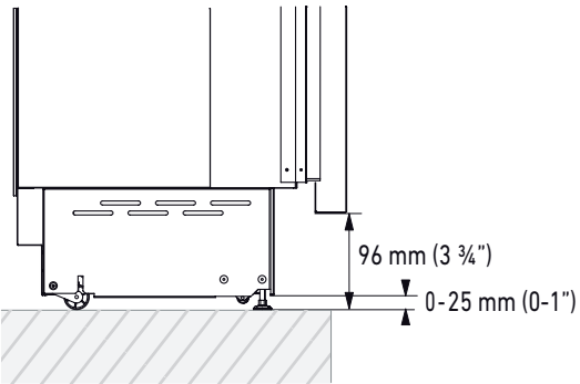
PLINTH SIZE
