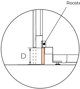
ROOSTER EN PLINT ZIJAAANZICHT
