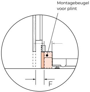
DIEPTE PLINT ZIJAAANZICHT
