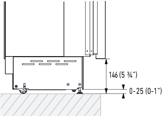
PLINTH SIZE
