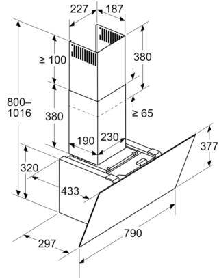
Afmeting in mm Apparaat in luchtcirculatiemodus
