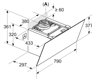
Afmeting in mm Apparaat in luchtcirculatiemodus zonder kanaal
