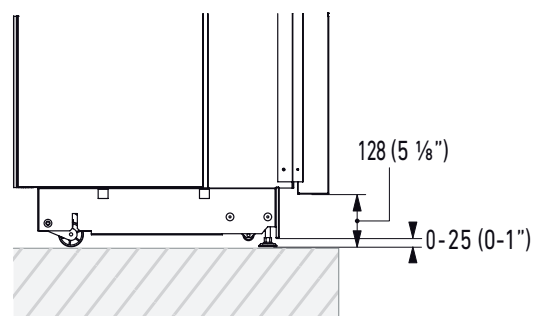
PLINTH SIZE
